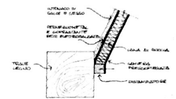
NODO 1 1:5
