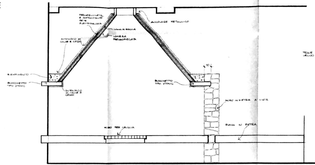
NODO 1 1:5
