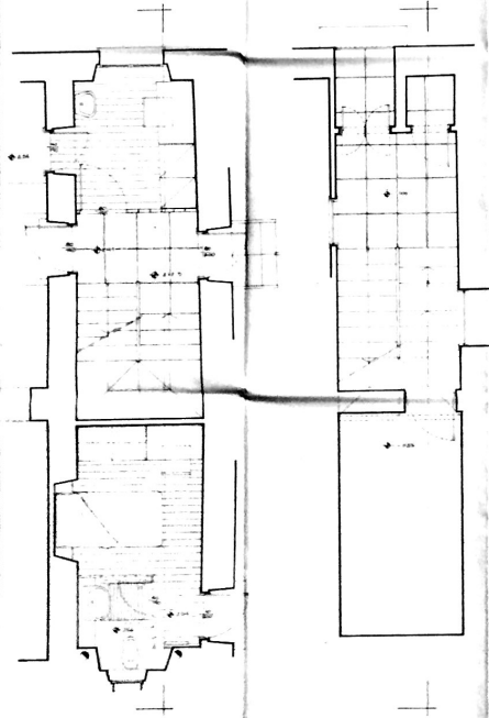
PIANO PRIMO
