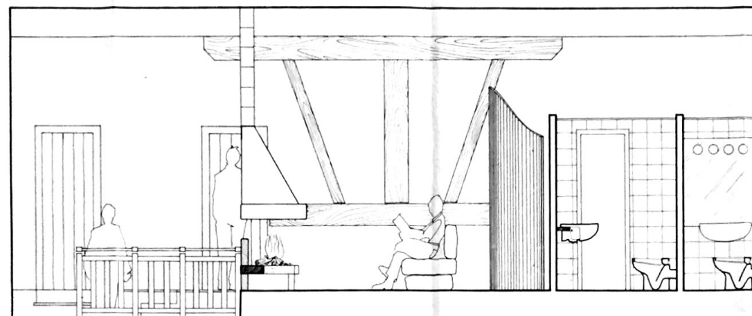
SEZIONE A-A
