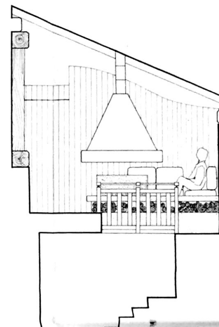
SEZIONE D-D
