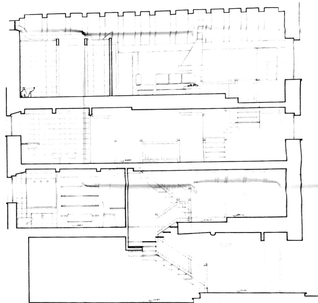
SEZIONE LONGITUDINALE
