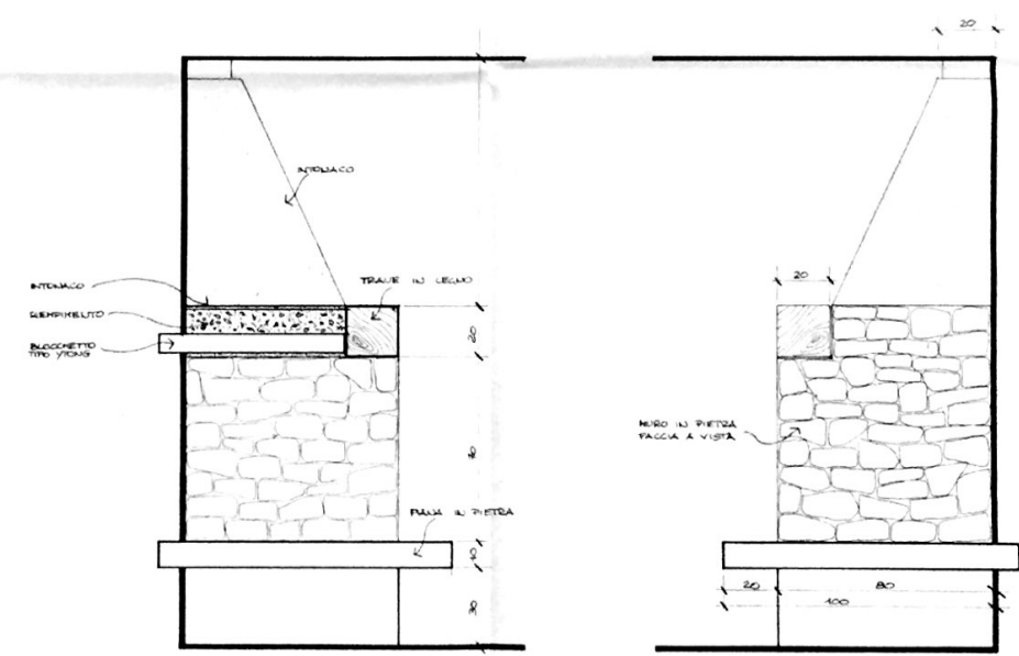
SEZIONE A-A' 1:10
