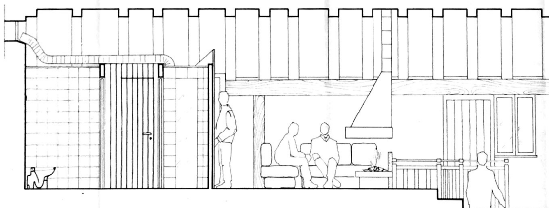
SEZIONE B-B
