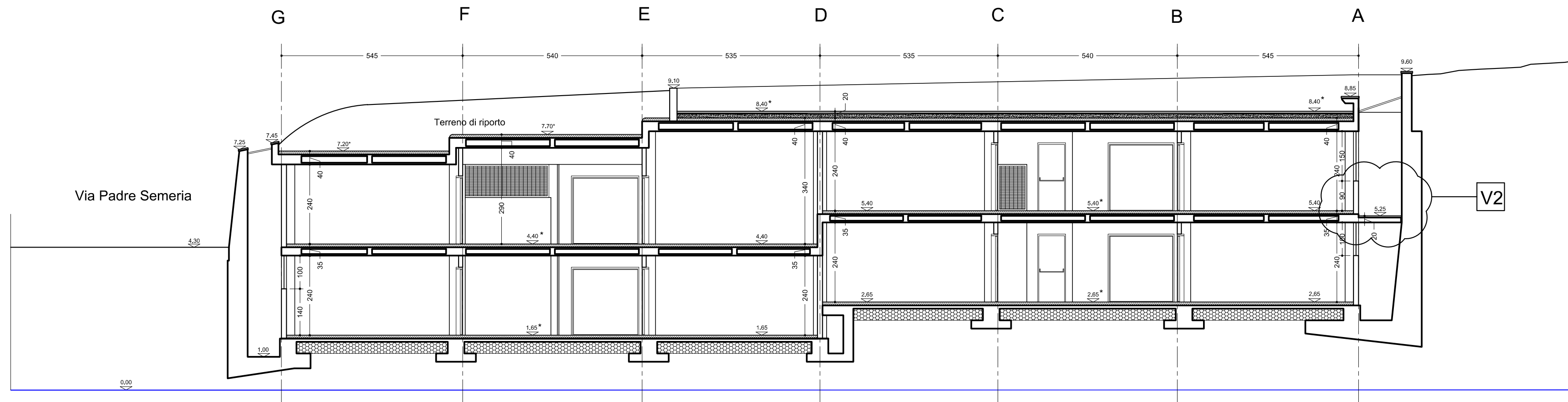
SEZIONE 3-3
