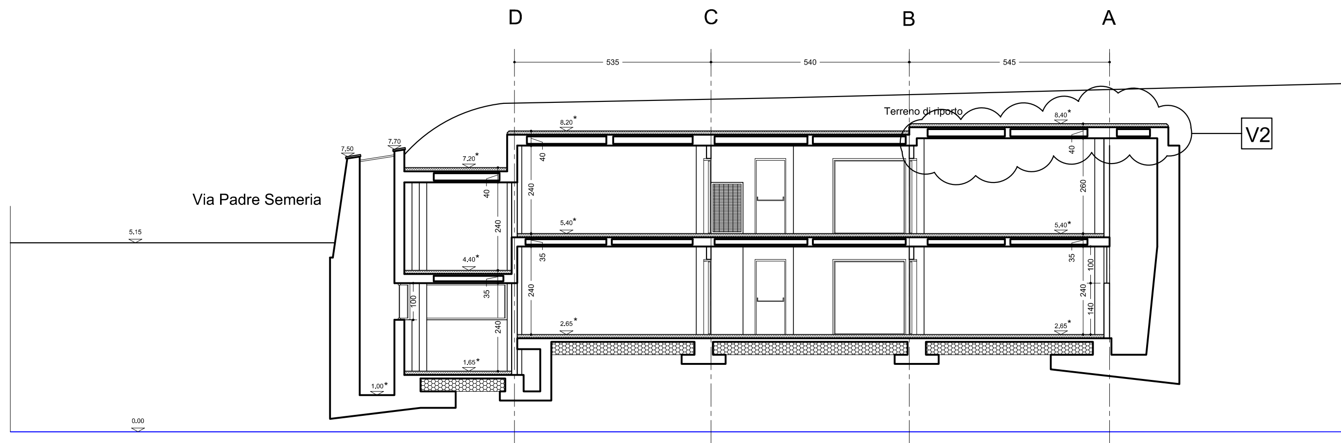
SEZIONE 4-4
